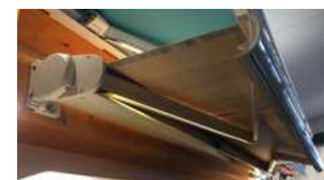
Bras testés à 20 000 cycles dotés d'une articulation à double câble gainé.
