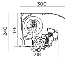
Perle et Perle Lux Pose Face avec auvent
