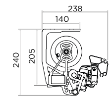
Perle et Perle Lux Pose Face
