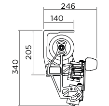
Jade bras croisés Pose Plafond
