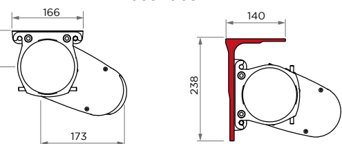
Ambre & Ambre Lux - Pose plafond -
