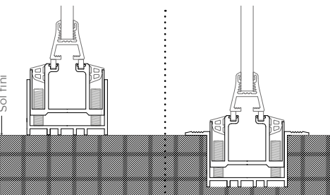
Rail posé au sol standard
