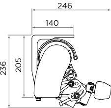
Jade Pose Plafond
