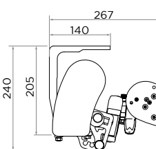
Perle Volant Pose Plafond
