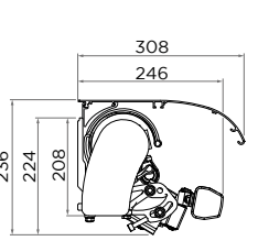
Jade avec auvent Pose Face
