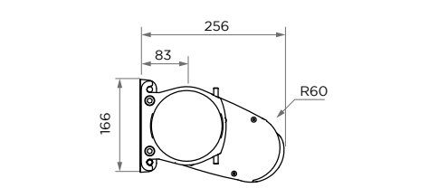
Ambre & Ambre Lux - Pose face -
