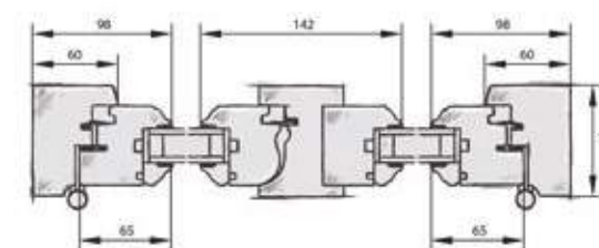
Coupe horizontale
