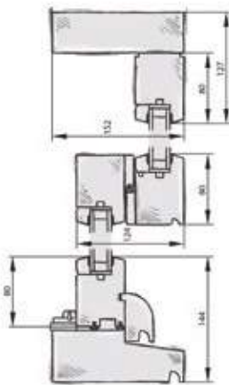
Coupe verticale
