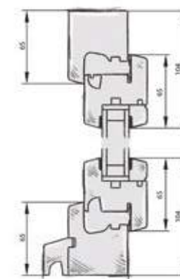
Coupe verticale
