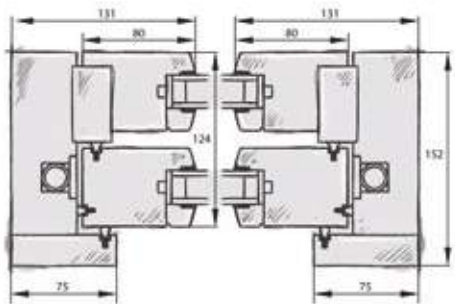
Coupe horizontale
