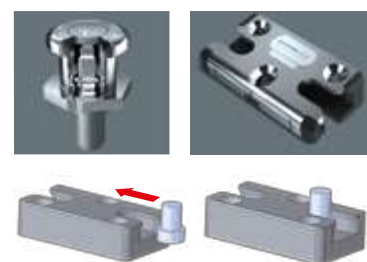
Rouleau KOPIBO et gâche de sécurité
