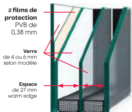
Triple vitrage
