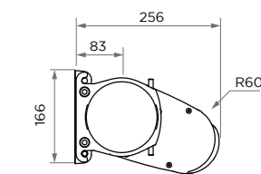
Ambre & Ambre Lux - Pose face -
