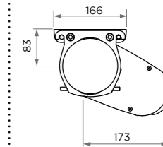
Ambre & Ambre Lux - Pose plafond -
