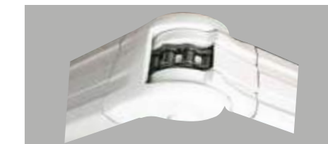
Bras testés à 60 000 cycles dotés d'une articulation chaîne à rouleaux.
