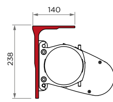
Ambre & Ambre Lux - Pose plafond avec equerre - 27
